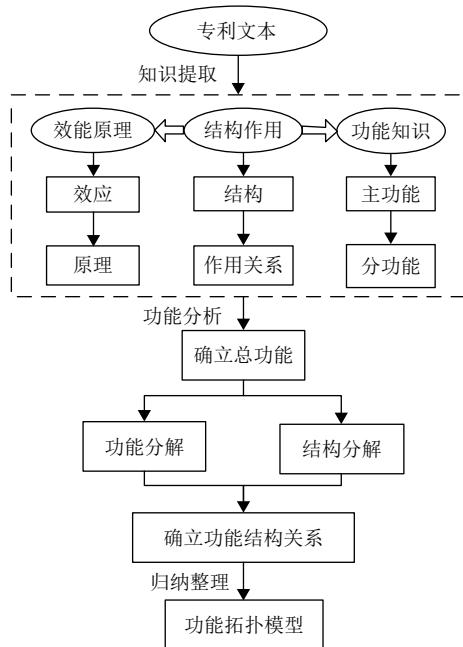
图2 专利知识功能模型建立流程
