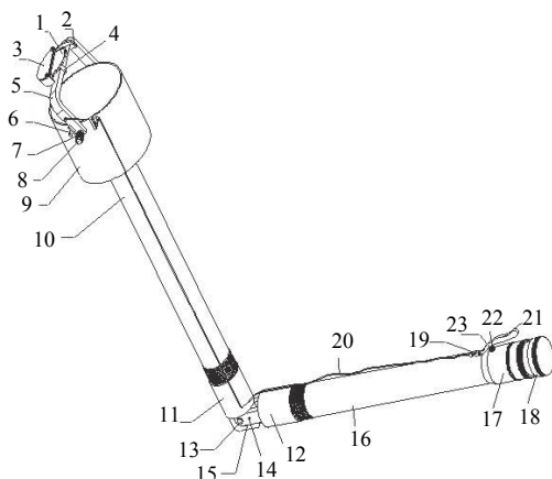
1-圆盘锯; 2-限位片; 3-防护罩; 4-电机; 5-U型支撑架; 6-限位凸台; 7-扭力弹簧; 8-销轴; 9-收集筐; 10-支撑杆A; 11-限位锁止装置A; 12-限位锁止装置B; 13-连接轴; 14-堵头螺钉; 15-限位孔; 16-支撑杆B; 17-控制把手; 18-端盖; 19-拉线; 20-套管; 21-按压柄; 22-按钮开关; 23-回位弹簧
