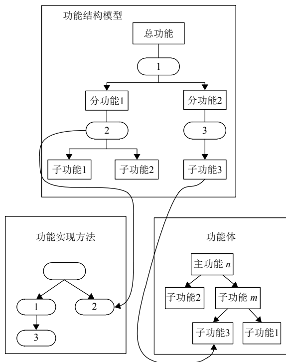
图1 功能本体体系结构关系图
